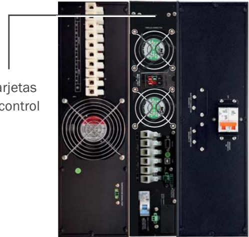
Transformador de aislamiento Módulo de control Banco de baterías
